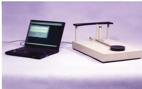
Рис. 1. Загальний вигляд приладу КВР-3.
